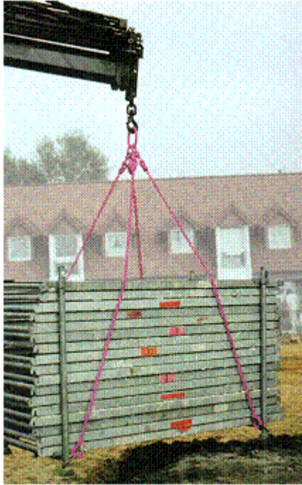
Abb. 200: Einsatz von Anschlagketten
