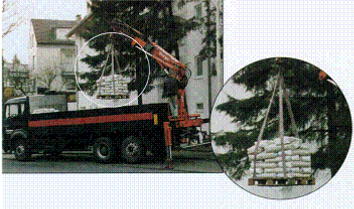
Abb. 240: Teile der Last sind nicht gegen Herabfallen gesichert
