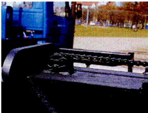
Abb. 30: Einzugstelle an ungesichertem Kettentrieb
