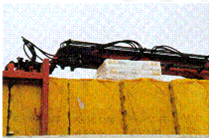
Abb. 273: Ungeeignet: Festklemmen von Teillasten zwischen Ausleger und Ladung
