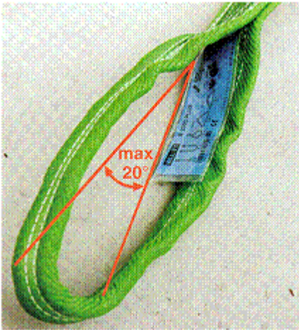
Abb. 210: Öffnungswinkel von Hebeband-Endschlaufen
