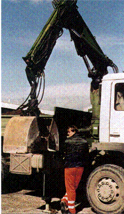
Abb. 65: Gefährlich: Bei der Flursteuerung muß sich der Kranführer im Gefahrenbereich des Auslegers aufhalten
