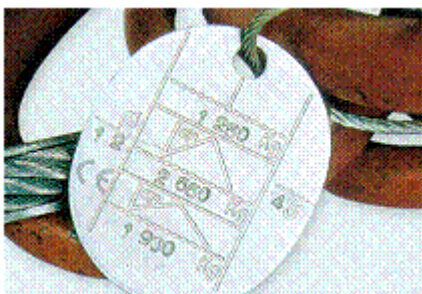
Abb. 218: Vorbildliche Tragfähigkeitsangabe auf einsträngigem Seil
