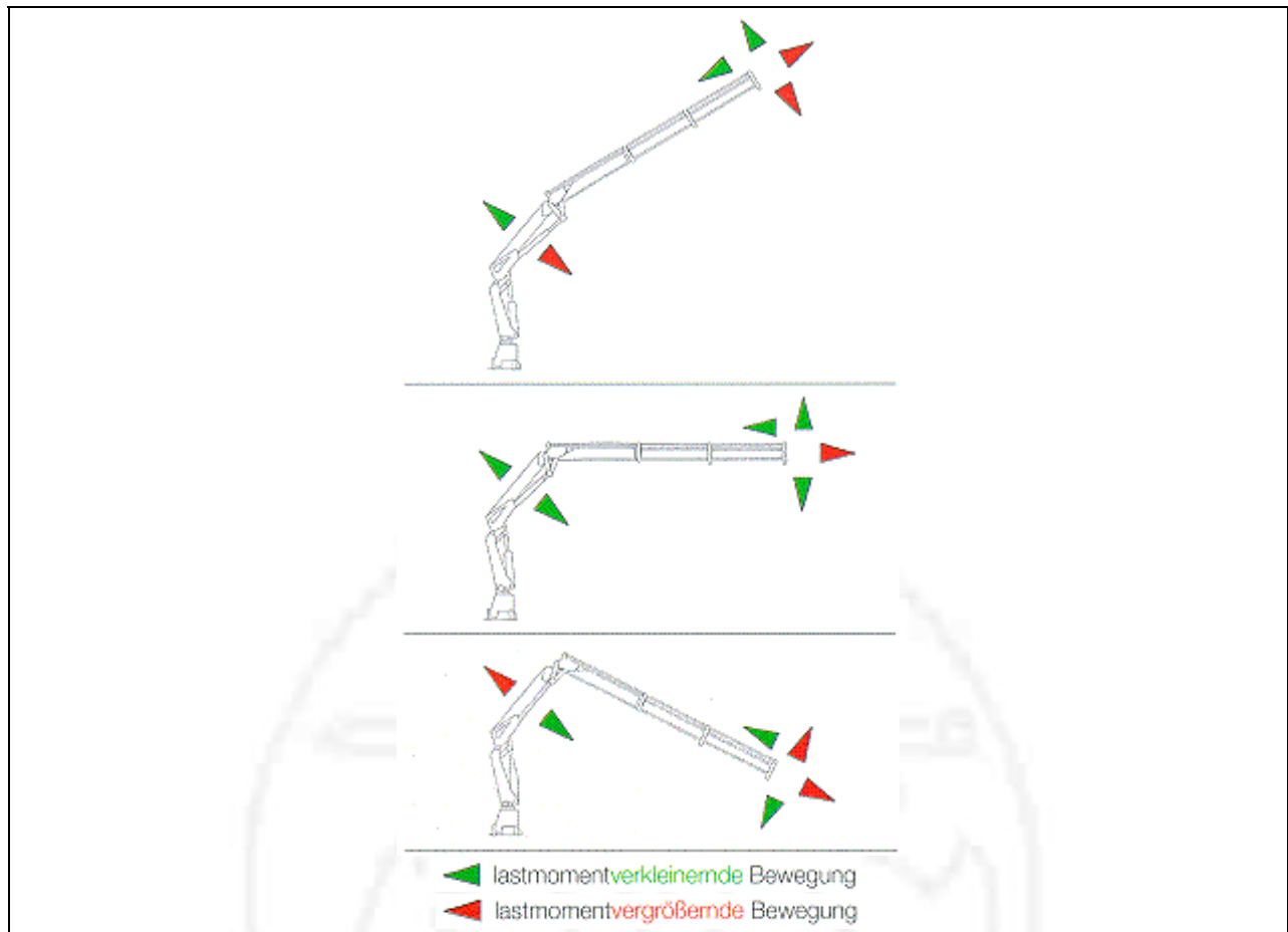
Abb. 106: Belastungskontrolle für Ladekran mit Knickausleger, sogen. SLC-System. Die Darstellung gilt nur für bereits freiehobene Lasten.
