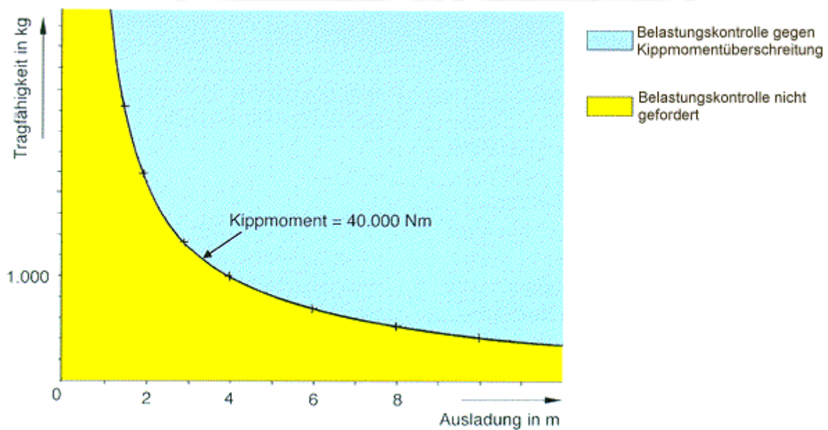
Abb. 103: Belastungskontrolle gegen Kippmomentüberschreitung
