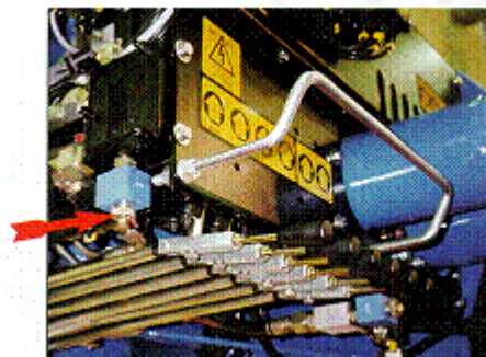
Abb. 111: Unzulässiger Überbrückungsschalter
