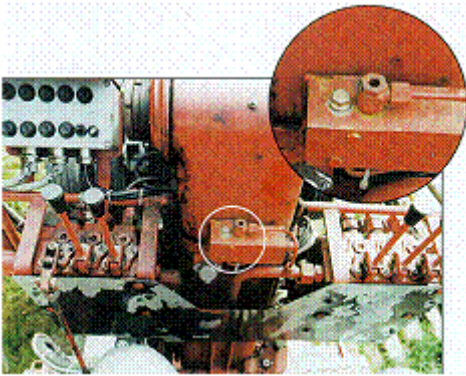
Abb. 169: Durch Schraube "blind" geschalteter Lastmomentbegrenzer
