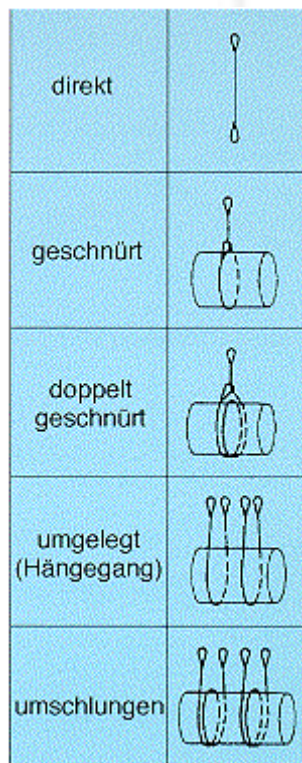
Abb. 235: Anschlagarten
