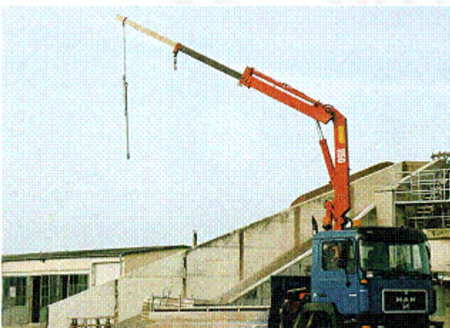
Abb. 116: Nicht zulässig: Verwenden ungeeigneter Schubstückverlängerungen
