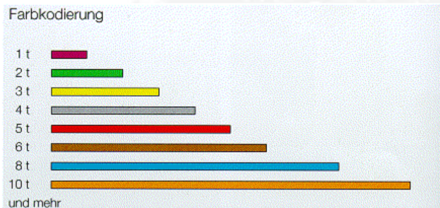
Abb. 209: Farbkodierung bei Hebebändern als optischer Hinweis auf die Tragfähigkeit
