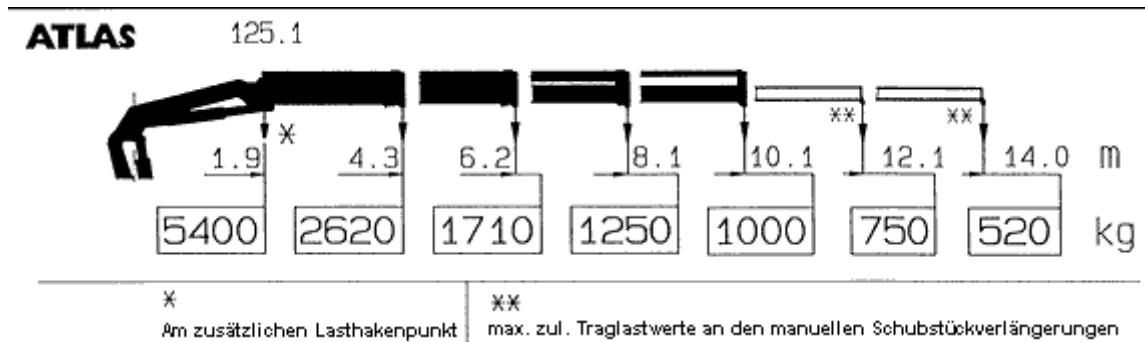
Abb. 93: Tragfähigkeitsdiagramm am Kran
