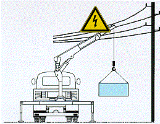
Abb. 178: Achtung! Stromübertritt bei Berühren oder Annähern
