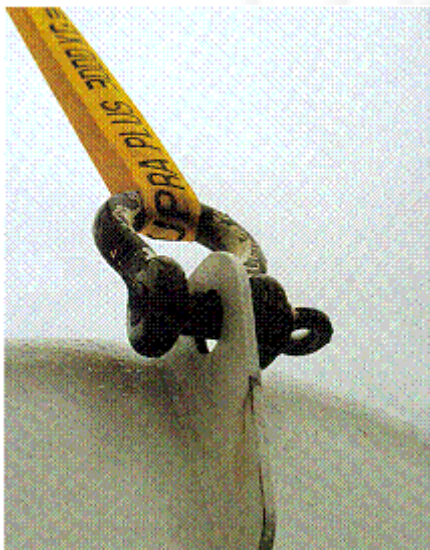
Abb. 254: Anschlagpunkte müssen einwirkende Kräfte sicher aufnehmen können
