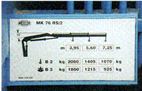
Abb. 132: Zulässige Tragfähigkeiten in Abhängigkeit von der Beanspruchungsgruppe
