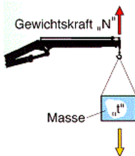
Abb. 12: Masse, Gewichtskraft
