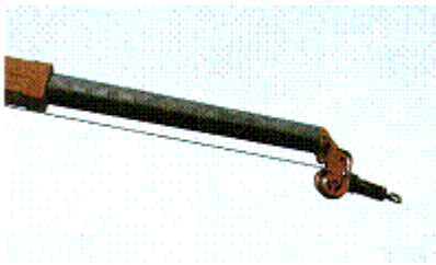
Abb. 96: Gefahr des Hubseilrisses durch fehlenden Hubendschalter
