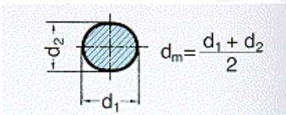
Abb. 263: Gemittelte Glieddicke
