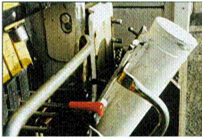
Abb. 154: Schraubenbruch durch Abstützfehler
