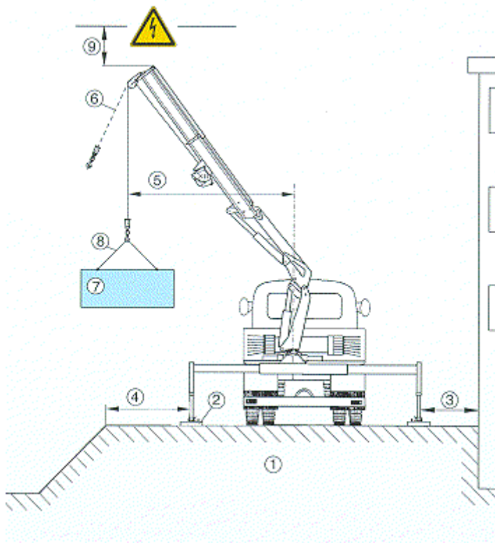
Abb. 139: Checkliste für Kранаufstellung
