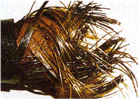
Abb. 46: Geplatzte Hydraulik-Schlauchleitung
