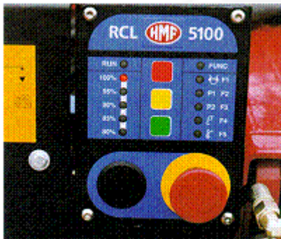
Abb. 112: Optische Warnung bei Erreichen der max. Tragfähigkeit
